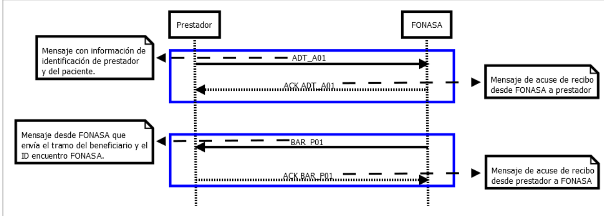
Imagen 3 Diagrama de secuencia para mensajería Validación
